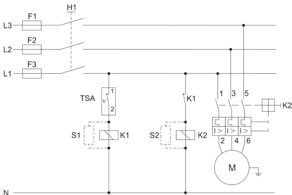
图1: 电路示例
