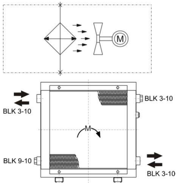
标准规格 BLK 1. 3 至 BLK 10
