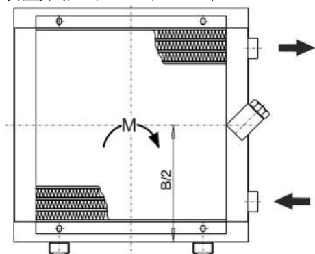
内置旁路 IB/ ITB (BLK 3-9)
