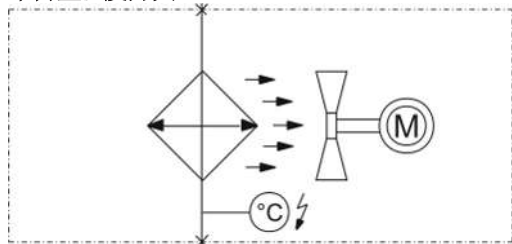
带内置温度开关
