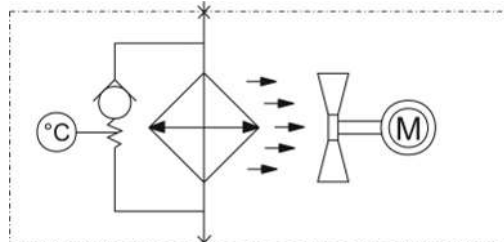
带温控旁通阀
