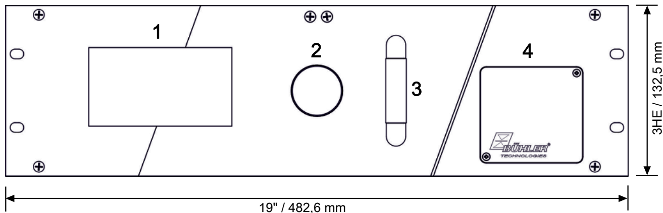
图 1: BA3MA, 前视图
