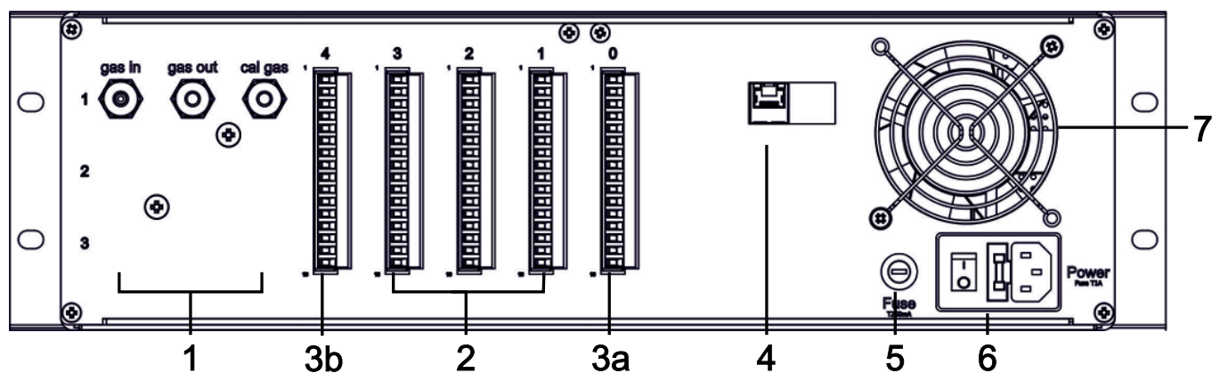
图 2: BA3MA, 后视图
