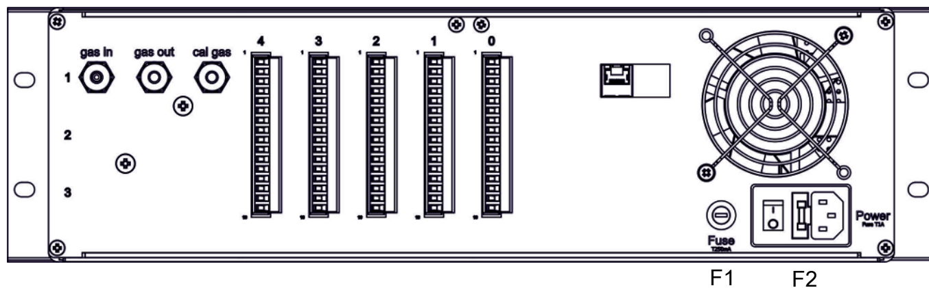
图 6: BA3 MA，后视图 保险丝
