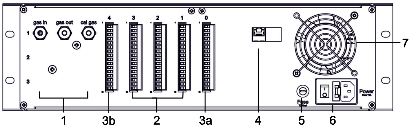
图 3: BA3MA, 后视图
