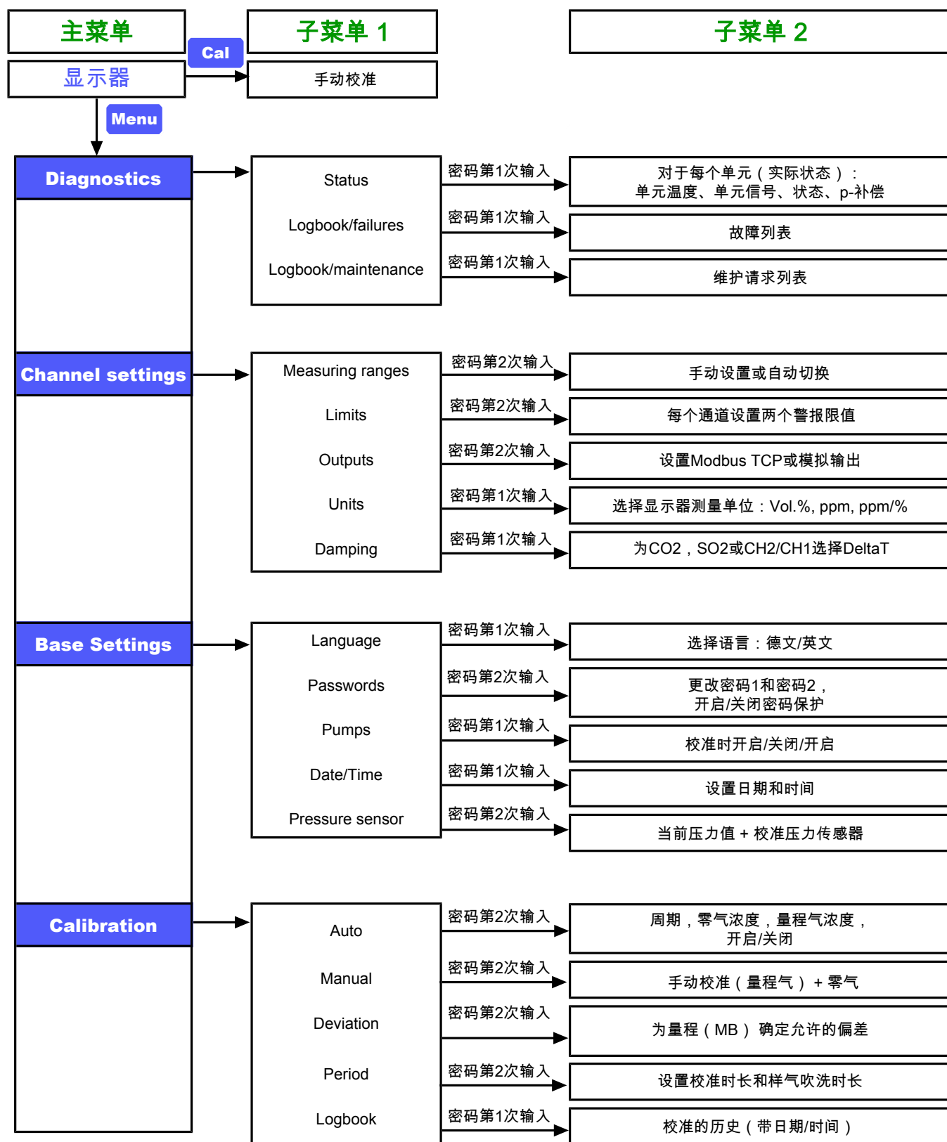
图 4: BA 3 MA菜单概览
