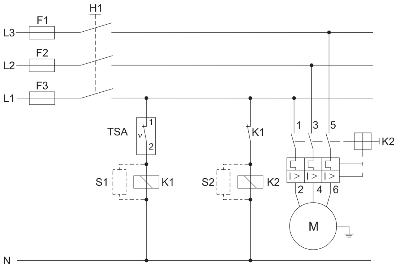
Fig. 1: Exemple de commutation
