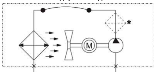
Стандартная модель
