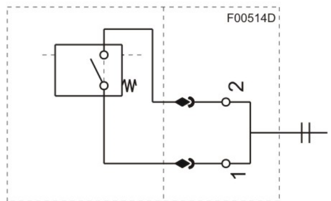
Abb. 2: Anschlussbelegung für Typ Mahle PIS 3085/2,2
