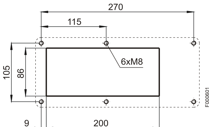
图1: 安装孔MT的孔图
