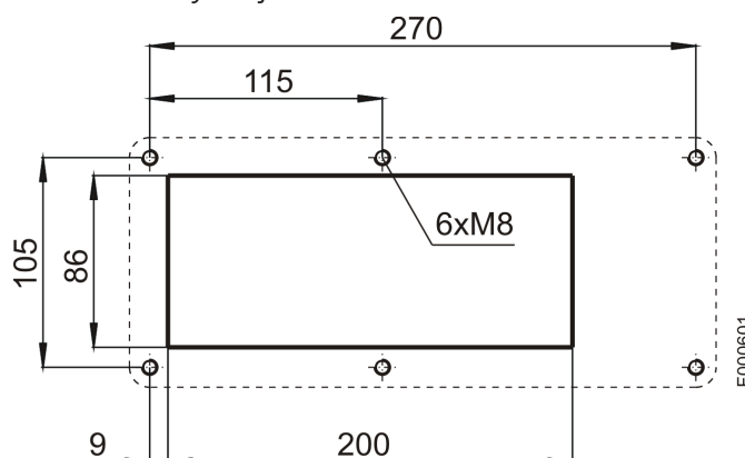
Ilus. 1: Patrón de orificios para la abertura de instalación MT
