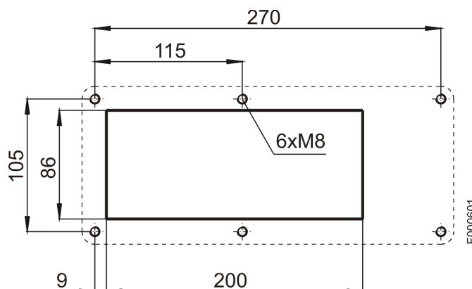
Fig. 1: Perforation pour l'ouverture de montage MT
