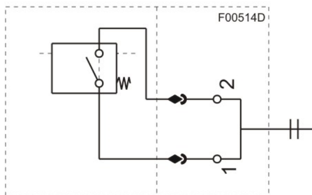
Ilus. 2: Disposición de conexiones para modelo Mahle PIS 3085/2,2
