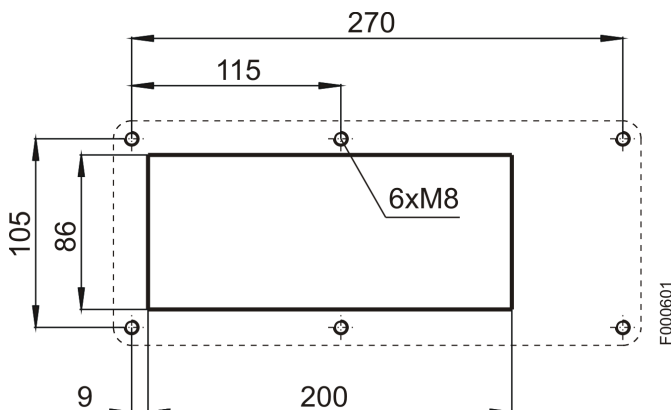
Изображение 1: Схема для монтажного отверстия МТ
