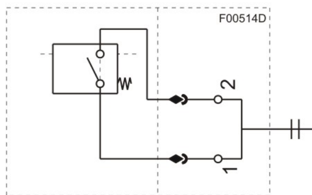
Fig. 2: Affectation des contacts pour le type Mahle PIS 3085/2,2
