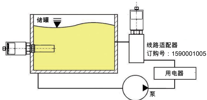
图1: 安装选项
