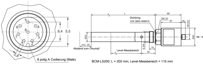
Anschlussmaße BCM-LS200
