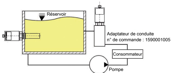
Fig. 1: Option d'installation
