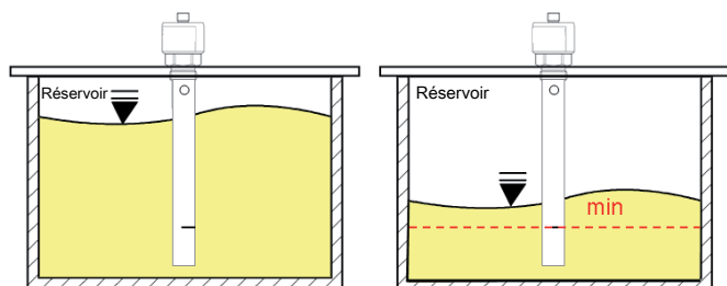
Fig. 2: Option d'installation
