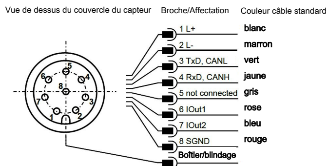
Fig. 4: Affectation des broches fiche du capteur
