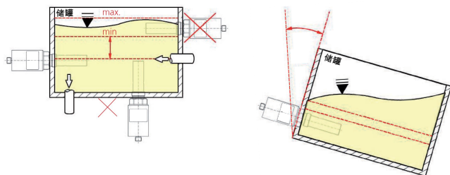
图3: 安装推荐
