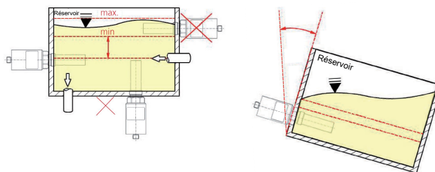
Fig. 3: Recommandations en matière d'installation
