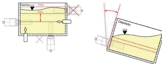
Ilus. 3: Recomendaciones de montaje
