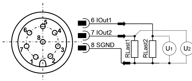
Изображение 6: Подключение нагрузочных резисторов для измерения аналоговых выходов 4..20 мА
