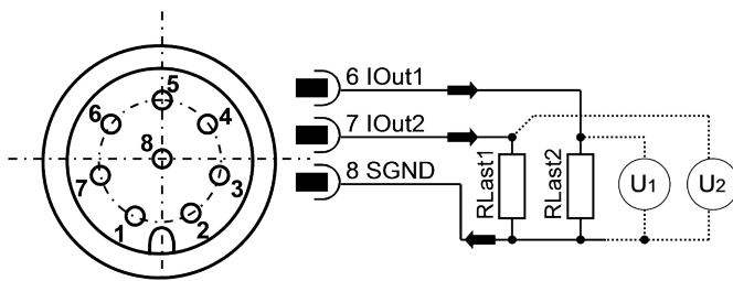
图6: 连接负载电阻以测量4...20 mA模拟输出
