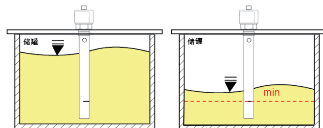
图2: 安装选项
