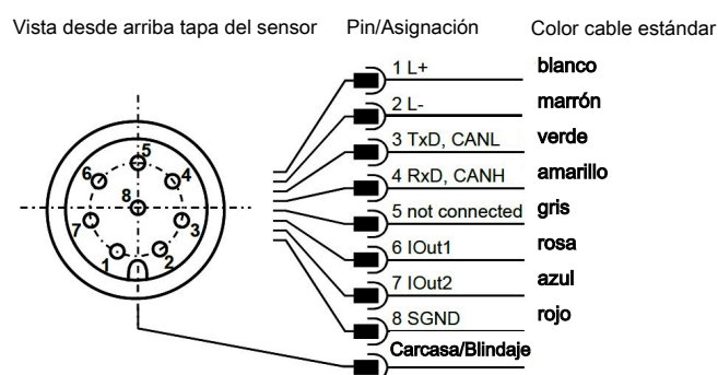
Ilus. 4: Asignación de pines conector de sensor
