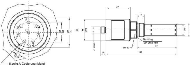
Anschlussmaße BCM-LS200
