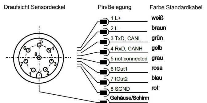
Abb. 4: Pinbelegung Sensorstecker
