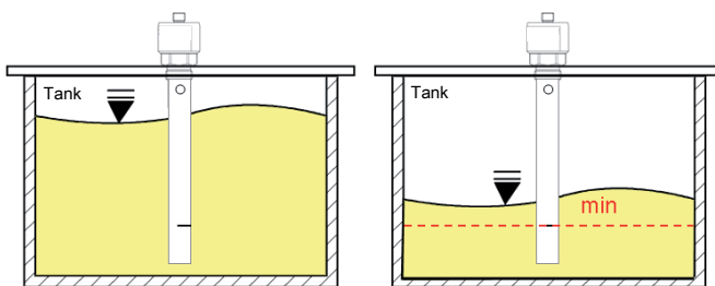
Abb. 2: Einbauoptionen
