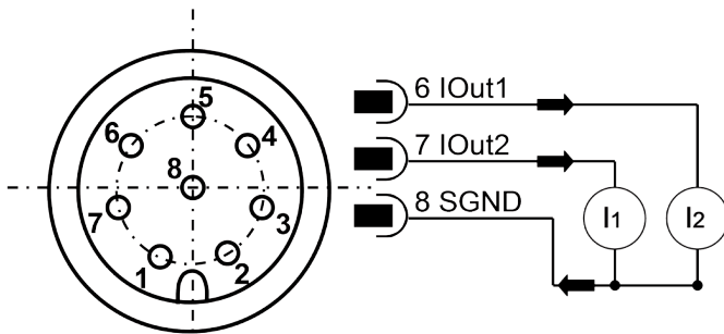
Abb. 5: Vermessung der analogen 4...20 mA Ausgänge ohne Lastwiderstände
