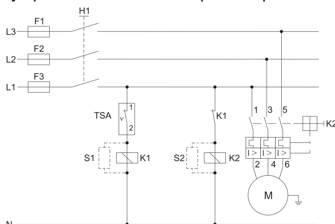
Ilustración 1: Ejemplo de conmutación
