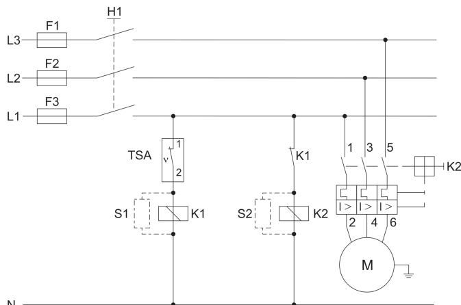
Abb. 1: Schaltungsbeispiel
