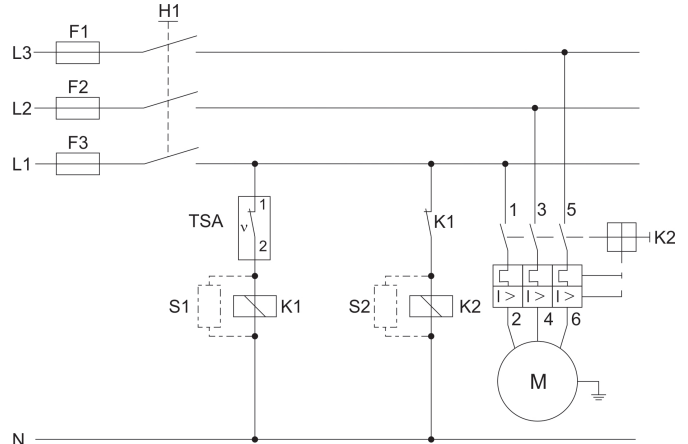
图1: 电路示例
