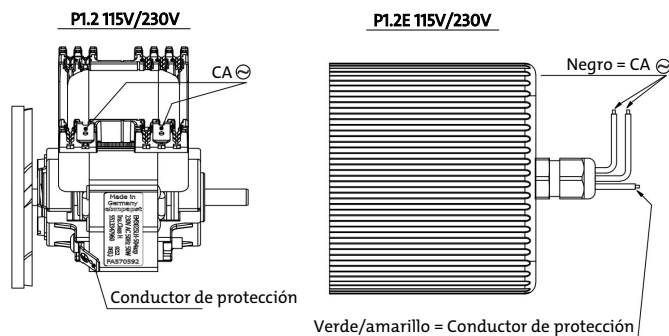
Ilus. 2: Conexiones eléctricas bombas P1.2
