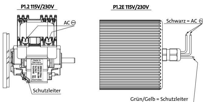
Abb. 2: Elektrische Anschlüsse P1.2 Pumpen
