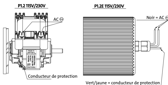
Fig. 2: Raccordements électriques de pompes P1.2
