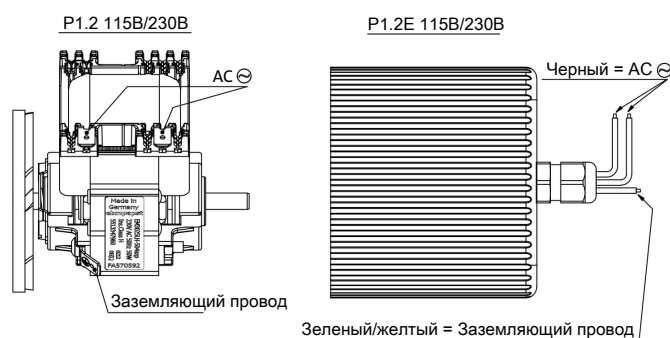
Изображение 2: Электрические подключения насосов P1.2
