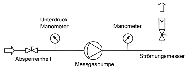
Abb. 1: Beispiel Flussschema einer geeigneten Überwachung
