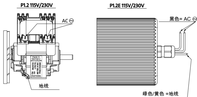
图2: P1.2泵的电气连接
