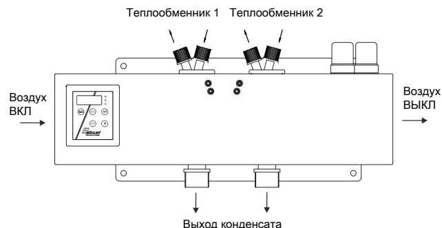
Схема потока:
