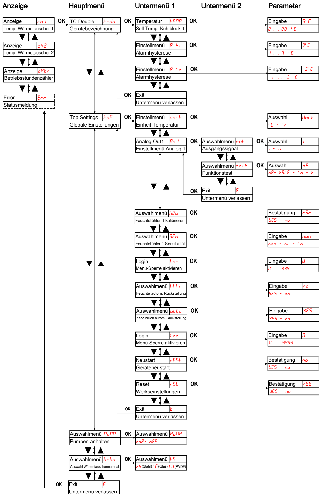
Abb. 1: Menüübersicht TC-Double
