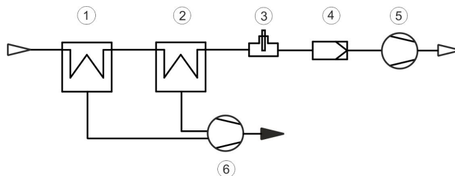
Схема потока:
