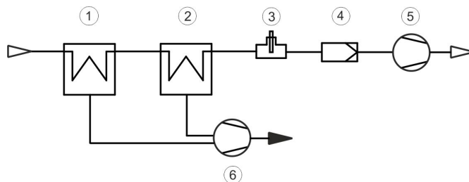
Flussplan:
