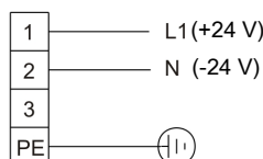
Raccordement secteur S1 115/230 V (24 V DC)
