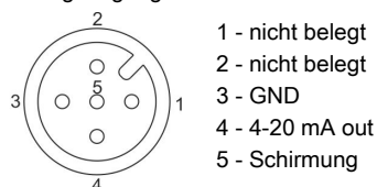
Analogausgang S3
