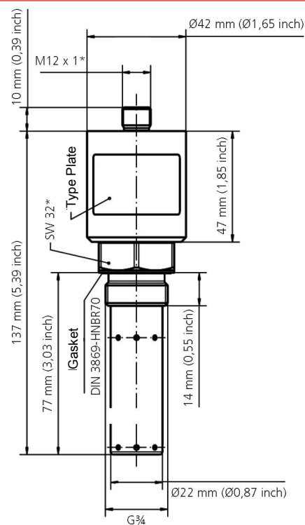
Dimensions
