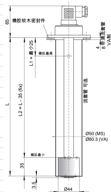
浮子SK 221
