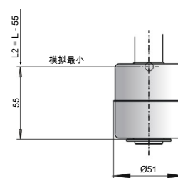
法兰图
