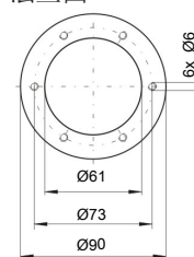
法兰图
