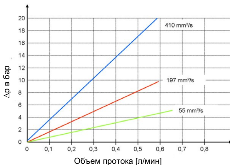
Изображение 1: Характеристика потока для различной вязкости без подключений Minimess
