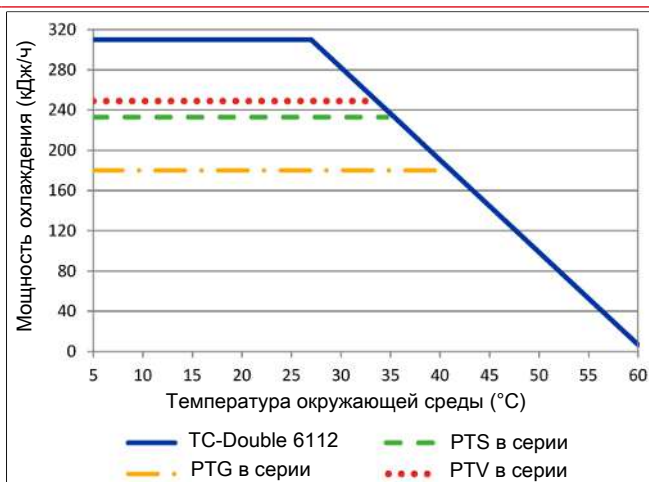
Тип TC-Double 6112
