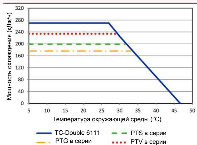
Тип TC-Double 6111
