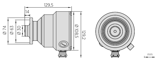
Abmessungen des PR53GC
