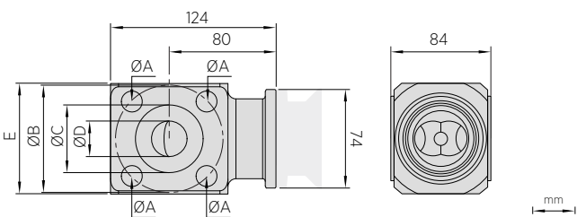
Wafer-Durchflussszelle FWFC mit Flansch
